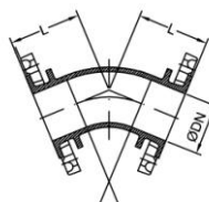
Joelho a Flange 45°
